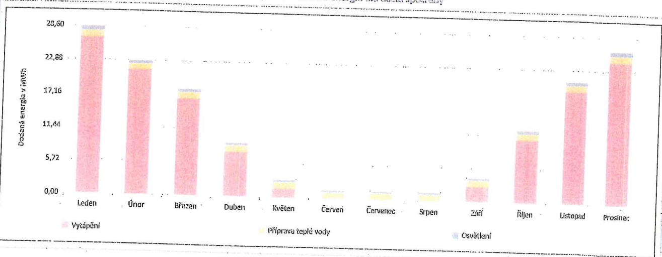
Roční průběh dodané energie dle účelů spotřeby
